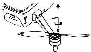
逆时针拧动螺丝，拆下螺旋桨。
